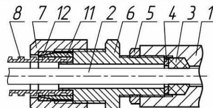
монтаж кабелем в металлорукуве KB15
