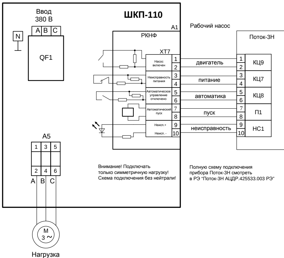
Рисунок 3. Схема электрическая подключения шкафа при эксплуатации
