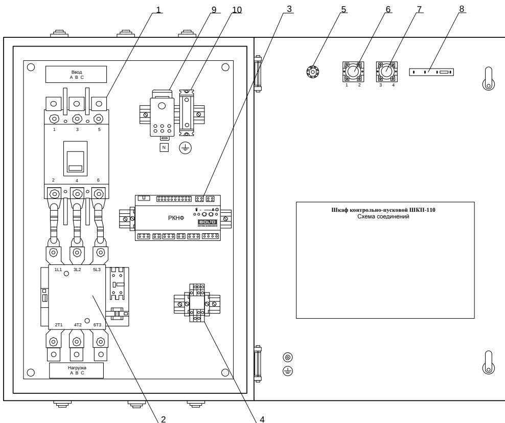
Рисунок 2. Внутреннее устройство шкафа
