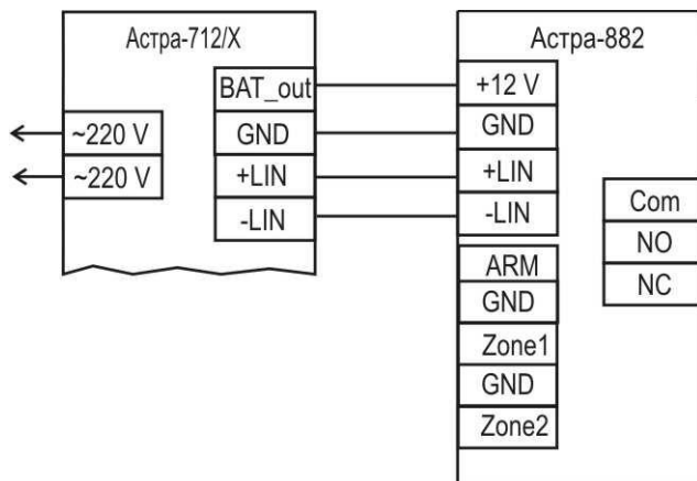
Рисунок 7 - Схема подключения ППКОП «Астра-712/Х» в расширенном режиме работы коммуникатора
