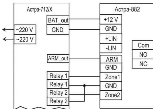
Рисунок 5 - Схема подключения ППКОП «Астра-712/Х» в автономном режиме работы коммуникатора
